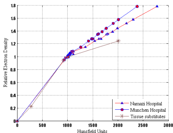
شکل ۲- منحنی چگالی الکترونی برحسب CT-number برای بافت های مختلف بدن با استفاده از روش استویکیومتری و مقایسه نتایج بدست آمده در بیمارستان نمازی و بخش فیزیک پزشکی دانشگاه مونیخ [۷]
