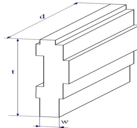
شکل ۷- یک تیغه کولیماتور چند تیغه‌ای
