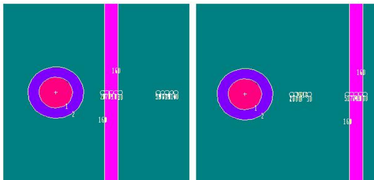
شکل ۳- هندسه‌ی شبیه‌سازی شده‌ی یک چشمه‌ی فعال در فانتوم ناهمگن
