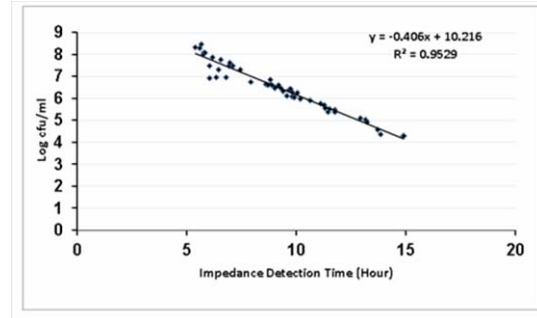
شکل ۱: منحنی ارتباط زمان‌های به دست آمده از دستگاه امیدانس با مقادیر بار باکتریایی شیر خام
