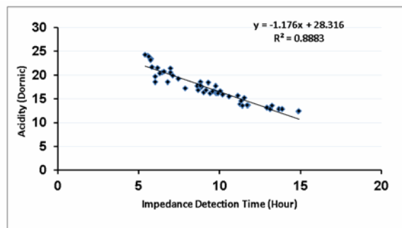
شکل ۳: منحنی ارتباط زمان‌های به دست آمده از دستگاه امیدانس با درجه دورنیک در شیر خام
