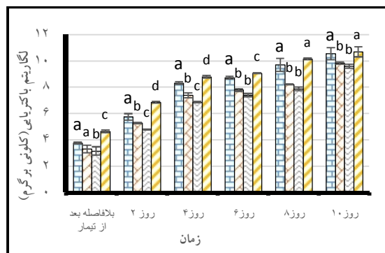
نمودار ۲: تغییرات میانگین و انحراف معیار شمارش باکتری‌های سایکروفیلیک در ۴ درجه‌ی سانتی‌گراد در ۴ گروه تیماری
