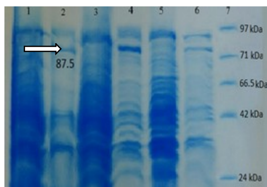
تصویر ۲: بررسی بیان پروتئین نوترکیب MBP-N با SDS-PAGE
