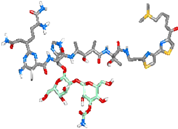
شکل ۱- ساختار فضایی آنتی‌بیوتیک بلئومایسین.
