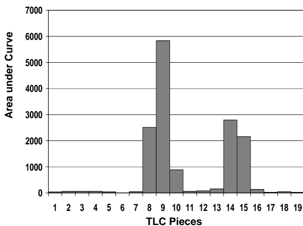
شکل ۳- رادیوکروماتوگرام محلول نشاندار شده کبالت-۵۷ بلئومایسین بر اساس پیک ۱۲۲ keV.
