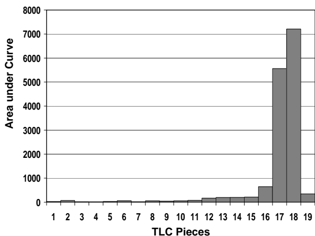
شکل ۲- رادیوکروماتوگرام محلول کبالت-۵۷ شسته شده با اسید کلریدریک بر اساس پیک ۱۲۲ keV.
