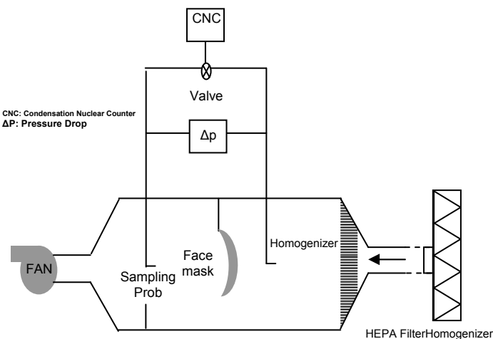
شکل ۱- نمای از تونل تست ماسک.
