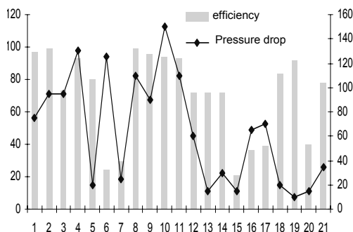
شکل ۴- افت فشار و کارایی ماسک‌های یکبار مصرف.
