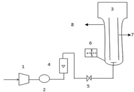
شکل ۱. طرح‌واره‌ی سیستم به کار رفته در آزمایش‌های فروشویی میکروبی؛ (۱) کمپرسور، (۲) صافی هوا، (۳) جداکننده‌ی گاز-مایع، (۴) جریان‌سنج، (۵) شیر کنترل، (۶) پخش‌کننده‌ی هوا، (۷) بالابر، (۸) زیست رآکتور.
