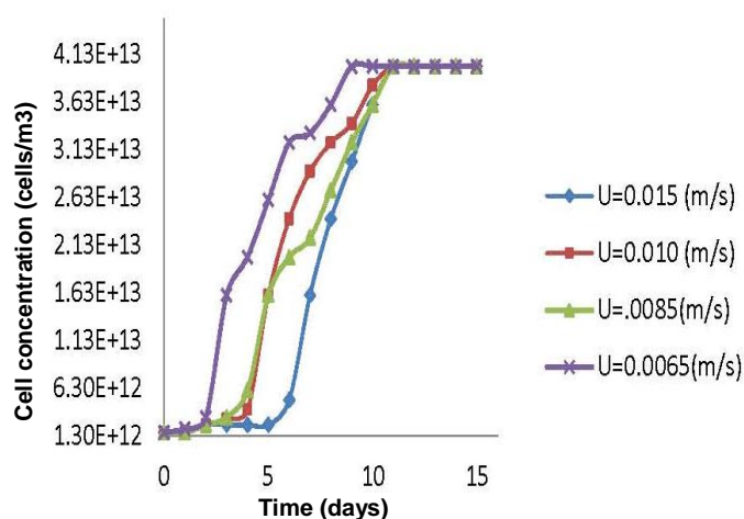
شکل ۶. تغییرات زمانی غلظت باکتری در سرعت‌های مختلف هوادهی.
