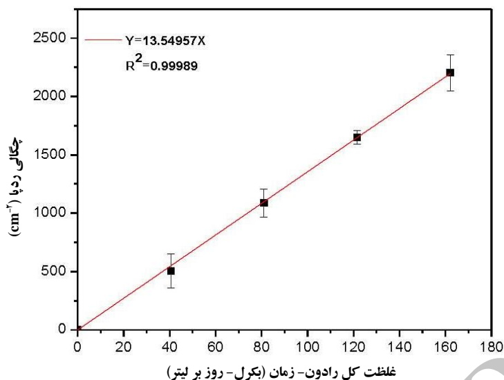
شکل ۴. منحنی پاسخ اتاقک نفوذی رادون پرتودهی شده.
