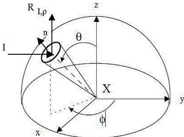
شکل ۴. پرتو تابشی I و بازتابشی R در مختصات کروی.
