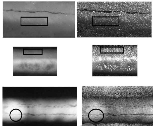
شکل ۵. نمونه‌هایی از نتیجه‌های حاصل از بازسازی تصویر با استفاده از روش استخراج شکل از سایه: سمت چپ تصویرهای پرتونگاری عیب‌ها و سمت راست تصویرهای بازسازی شده‌ی عمق.
