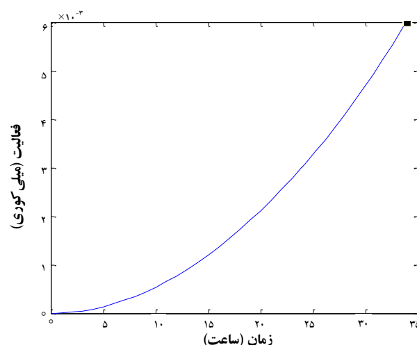
شکل ۳. تغییر زمانی فعالیت ترییم-۱۶۱ حاصل از پرتودهی ۱ میلی گرم ترییم طبیعی با شار نوترون گرمایی 3 \times 10^{13} \text{ cm}^{-2} \text{ s}^{-1} .
