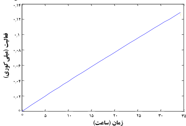
شکل ۴. تغییر زمانی فعالیت ترییم-۱۶۰ حاصل از پرتودهی ۱ میلی گرم ترییم طبیعی با شار نوترون گرمایی 3 \times 10^{13} \text{ cm}^{-2} \text{ s}^{-1} .
