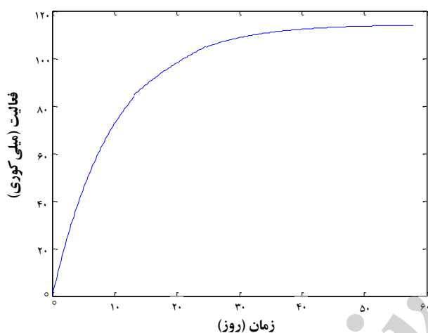
شکل ۷. تغییر فعالیت ترسیم-۱۶۱ حاصل از پرتودهی ۱۰ میلی گرم گادولینیم-۱۶۰ (۹۸٫۲٪ غنی شده) با شار نوترون گرمایی 8 \times 10^{13} \text{ cm}^{-2} \text{ s}^{-1} برحسب زمان.
