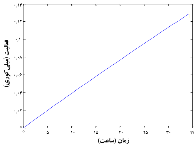
شکل ۵. تغییر فعالیت ترسیم-۱۶۱ حاصل از پرتودهی ۱ میلی گرم گادولینیم اکسید طبیعی در رآکتور با شار نوترون گرمایی 3 \times 10^{13} \text{ cm}^{-2} \text{ s}^{-1} برحسب زمان.
