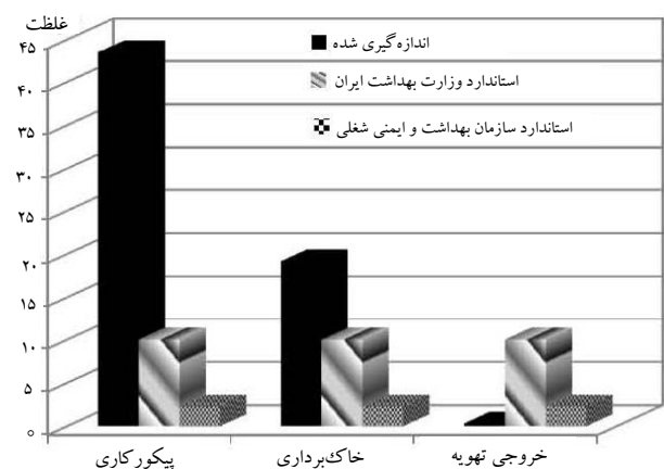
شکل ۱. مقایسه مقدار گردوغبار قابل‌تنفس با استاندارد وزارت بهداشت ایران و سازمان بهداشت و ایمنی شغلی.
