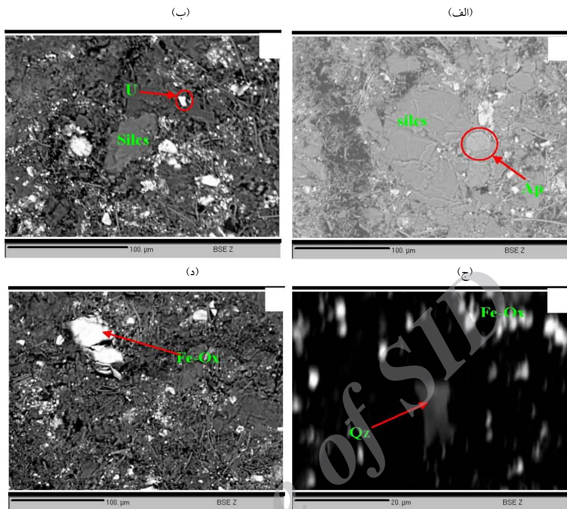
شکل ۶. ریزنگارهای الکترونی آبروسل‌های برداشت شده از محل پیکورکاری تونل. (الف) ذراتی از جنس آپاتیت و سیلیکات‌ها، (ب) ذراتی از جنس اورانیم و سیلیکات‌ها، (ج) ذراتی از جنس کوآرتز و اکسید آهن، (د) ذره‌ای از جنس اکسید آهن.
