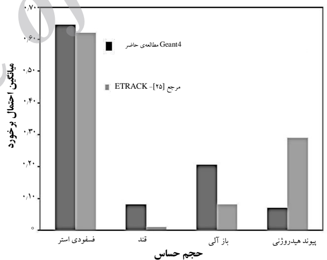
شکل ۳. میانگین احتمال برخورد برای انرژی‌های ۳، ۴.۵، ۸، ۱۰، ۱۴، ۱۷، ۲۰ کیلوالکترون‌ولت در هر یک از حجم‌های چهارگانه‌ی سازنده‌ی مدل B-DNA و مقایسه‌ی آن با داده‌های مرجع [۲۵]. برای گستره‌ی ۲۵۰ الکترون‌ولت تا ۲۰ کیلوالکترون‌ولت.
