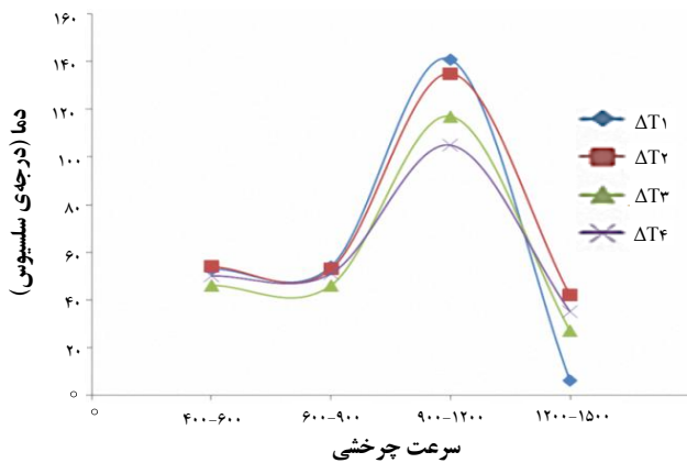
شکل ۳. رابطه‌ی بین دما و سرعت چرخشی.
