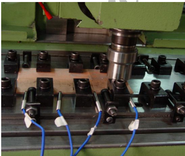
شکل ۲. موقعیت ترموکوپل‌ها در درون قطعه‌ی کار.
