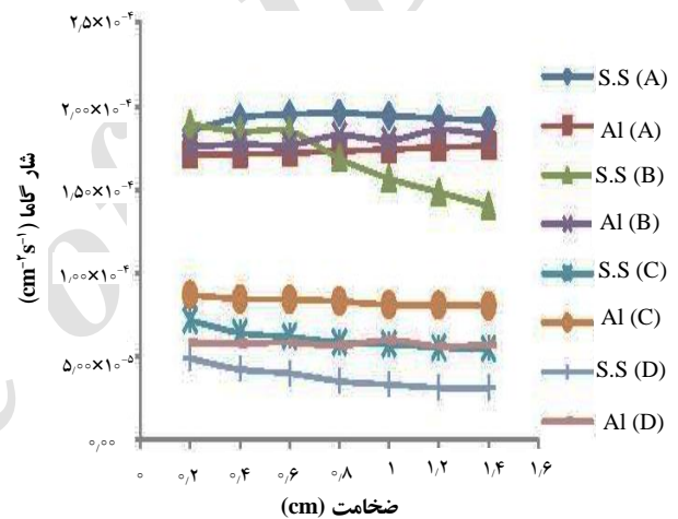
شکل ۴. رابطه‌ی بین شار گاما و ضخامت و جنس ماده‌ی دیواره‌ی باریکه‌ساز.
