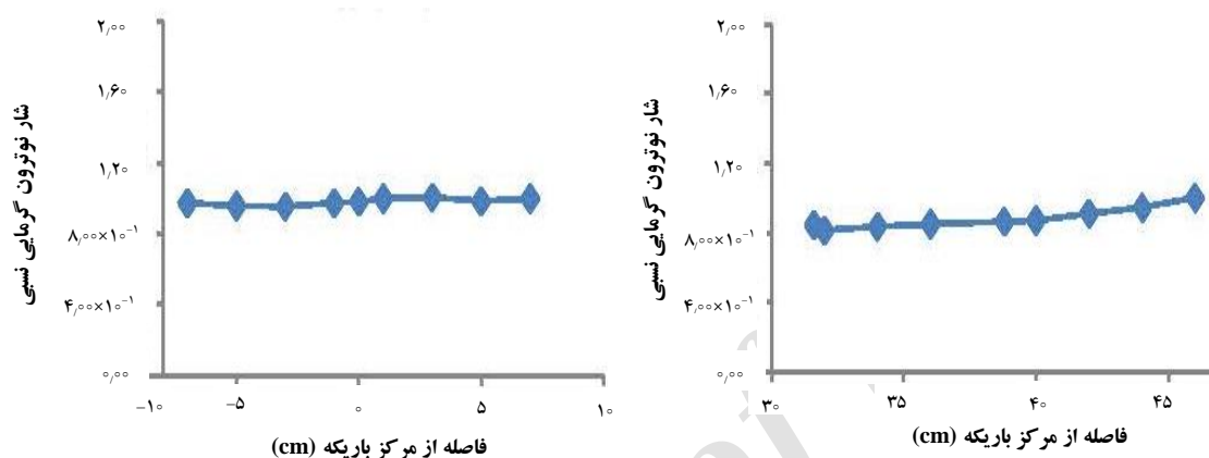
شکل ۸. الف) توزیع شار نوترون گرمایی بر روی محور Y = 0 برای X های مختلف نسبت به مرکز باریکه‌ساز؛ ب) توزیع شار نوترون گرمایی در خروجی باریکه‌ساز بر روی محور X = 38,801 (مرکز باریکه‌ساز) برای Y های مختلف.
