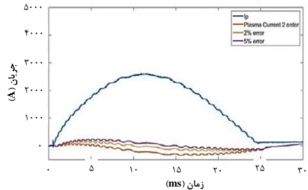
شکل ۱۰. جریان محاسبه شده توسط المان محدود مرتبه دوم با اعمال ۲ و ۵ درصد خطا به مقادیر اندازه‌گیری شده پروب‌های مغناطیسی و همچنین جریان اندازه‌گیری شده توسط پیچه روگوفسکی توکامک دماوند.
