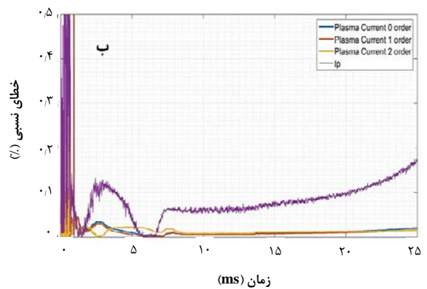
شکل ۹. خطای نسبی جریان اندازه‌گیری شده توسط پیچ‌ه روگوفسکی خارجی که در نمودار با I_p نشان داده شده است و جریان اندازه‌گیری شده توسط پیچ‌ه روگوفسکی داخلی با روش‌های محاسباتی مختلف (الف) پیچ‌های تعادلی و (ب) پیچ‌های اهمی روشن هستند.
