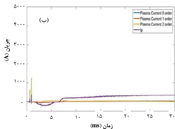
شکل ۸. جریان اندازه‌گیری شده توسط پیچه روگوفسکی خارجی ( I_p ) و جریان اندازه‌گیری شده توسط پیچه روگوفسکی داخلی با روش‌های محاسباتی مختلف الف) پیچه‌های تعادلی و ب) پیچه‌های اهمی.
