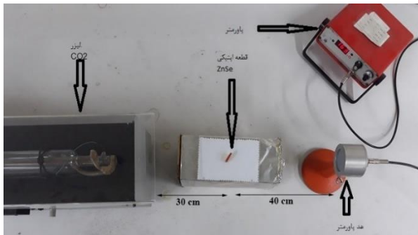
شکل ۴. نمایی از چیدمان لیزر و نمونه‌ها برای محاسبه میزان عبور.
