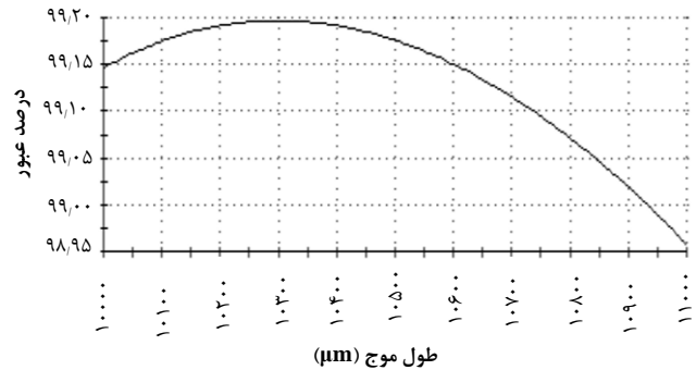
شکل ۲. میزان عبور پوشش ضدبازتاب طراحی شده بر حسب طول موج با استفاده از نرم‌افزار Macleod.
