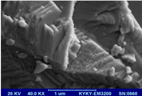
شکل ۶. آنالیز SEM مربوط به لایه نشانی ضدبازتاب بر روی \text{ZnSe}
