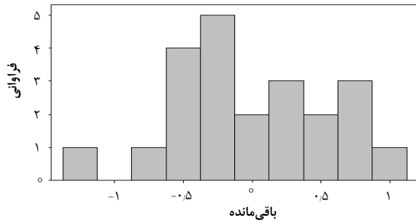
شکل ۳. هیستوگرام خطاهای باقی مانده.
