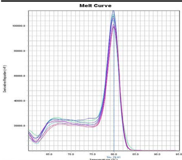
نمودار ۵. منحنی ذوب ژن BCL-XL با نقطه ذوب 79/91°C
