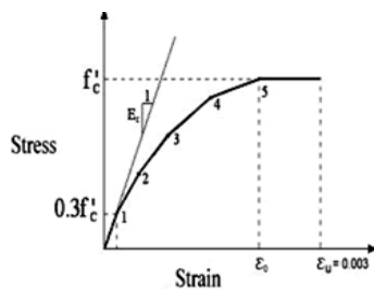
شکل ۲ رفتار الاستیک غیرخطی بتن در فشار [26]
