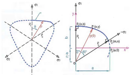
شکل ۳ منحنی شکست William-Warnke. [24]
