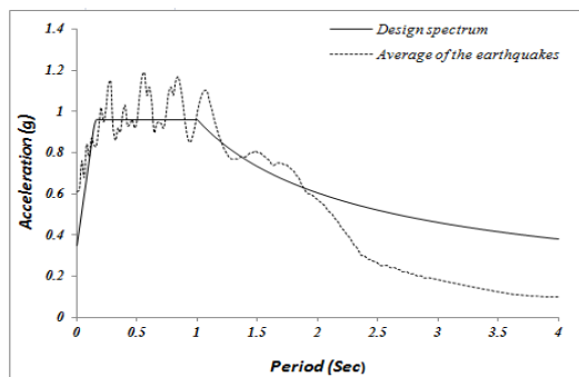
شکل ۴ طیف طرح و طیف میانگین رکوردهای زلزله‌ی نورتریج
