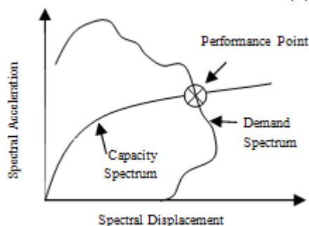
شکل ۱ نقطه‌ی عملکرد در روش طیف ظرفیت
