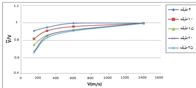
شکل ۱۷ نمودار نسبت های \frac{\bar{a}}{V} (برش پایه سازه ها) برای خاک های معرفی شده در سرعت های موج برشی مختلف
