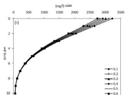
تأثیر تغییر تخلخل بر ماسه سنگ
