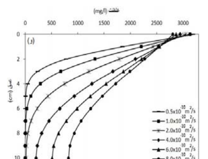
تأثیر تغییر ضریب انتشار مولکولی بر ماسه سنگ
