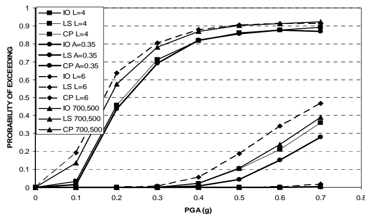
شکل ۲ منحنی‌های شکندگی قاب‌های ۳ طبقه با تنوع پارامترهای طراحی
