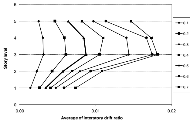
شکل ۸ تغییرات نسبت تغییر مکان مکان جانبی طبقات در شدت‌های مختلف برای قاب پنج‌طبقه مینا
