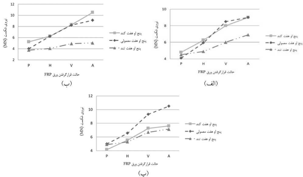
شکل ۱۲ نمودارهای تغییرات نیروی شکست در برابر حالت قرارگرفتن ورق FRP در حالت اعمال نیرو در یک سوم بالایی ارتفاع گنبدهای پنج و هفت دهانه‌های: الف) ۱۲m، ب) ۱۵m، پ) ۱۸m
