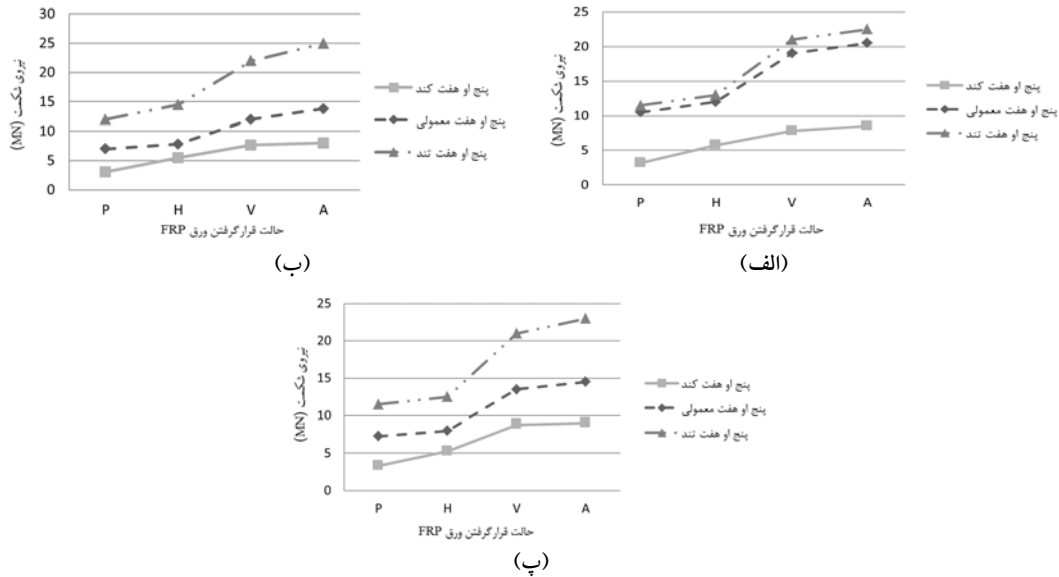
شکل ۱۴ نمودارهای تغییرات نیروی شکست در برابر حالت قرارگرفتن ورق FRP در حالت اعمال نیرو در یکسوم پایینی ارتفاع گنبدهای پنج و هفت برای دهانه‌های: الف) ۱۲m، ب) ۱۵m، پ) ۱۸m
