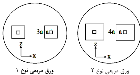
شکل ۸ نمای بالا از گروه ۳ چیدمان ورق‌های FRP در حالت دور تا دور ورق فولادی در دو حالت با ابعاد ۳ و ۴ برابر ابعاد ورق فولادی
