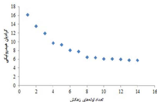
شکل ۲۲ تأثیر آرایش تعدادی لوله‌های زهکش در حالت بهینه بر گرادینان هیدرولیکی
