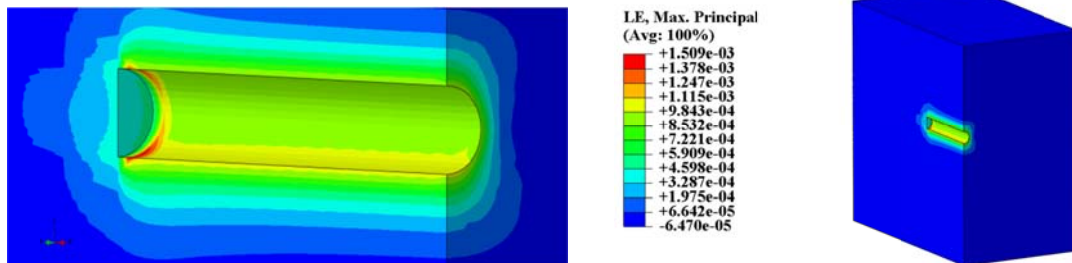
شکل ۸ کانتور کرنش ماکزیمم برای مدل پایه
