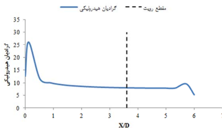
شکل ۱۱ گرادینان هیدرولیکی
