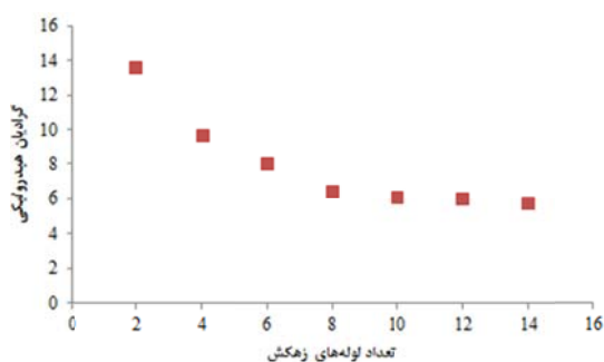
شکل ۲۳ تأثیر آرایش تعدادی لوله‌های زهکش در حالت زوج بر گرادینان هیدرولیکی
