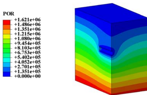
شکل ۱۰ کانتور فشار آب حفره‌ای برای مدل پایه (Pa)
