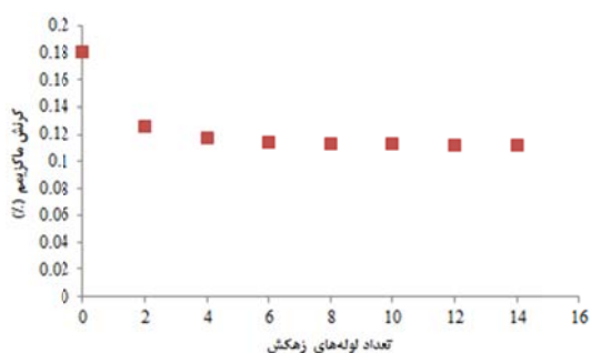
شکل ۲۵ تأثیر آرایش تعدادی لوله‌های زهکش در حالت زوج بر کرش ماکزیمم
