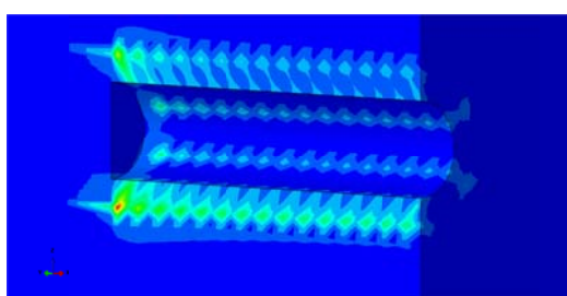
شکل ۱۲ کانتور گرادینان هیدرولیکی برای مدل پایه
