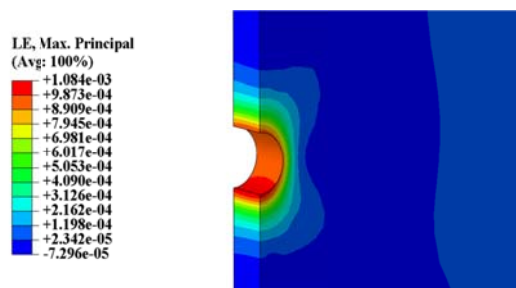
شکل ۳۸ کانتور کرنش ماکزیمم در آرایش بهینه سیستم زهکش چتری
