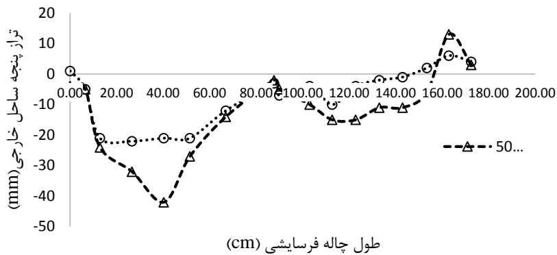
شکل ۱۰ تغییرات تراز بستر در پنجه ساحل خارجی در زوایای ۱۰ و ۲۰ درجه (۱۰-الف)، ۳۰ و ۴۰ درجه (۱۰-ب) و ۵۰ و ۶۰ درجه (۱۰-ج)
