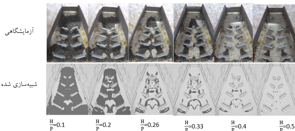
شکل ۷ الگوی رسوب‌گذاری در بالادست سرریز نوک اردکی: h_v = 0.07 m
