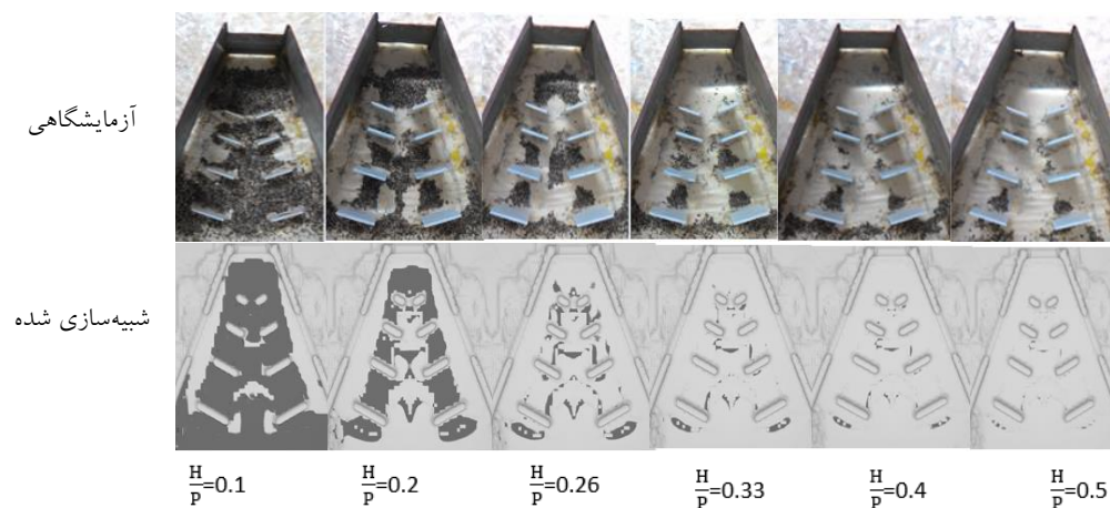
شکل ۸ الگوی رسوب‌گذاری در بالادست سرریز نوک اردکی: h_v = 0.1 m
