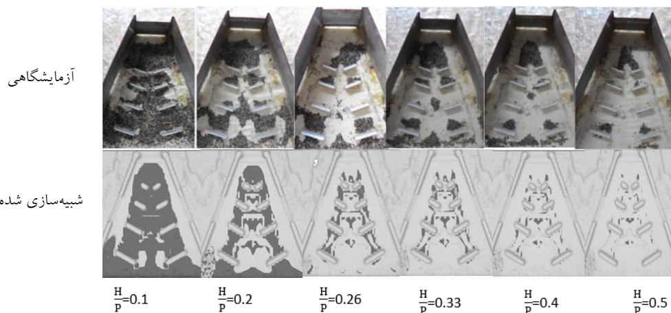
شکل ۶ الگوی رسوب‌گذاری در بالادست سرریز نوک اردکی: h_v = 0.04 m
