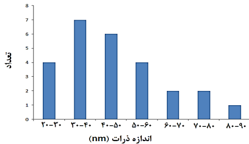
شکل ۱ منحنی اندازه نانوذرات اکسید سیلیسیم.
