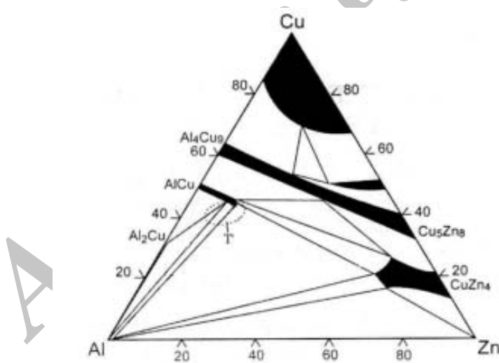
شکل ۸ مقطع همدمای دیاگرام فازی سه تایی روی-آلومینیوم-مس در دمای اتاق [۱۸]
