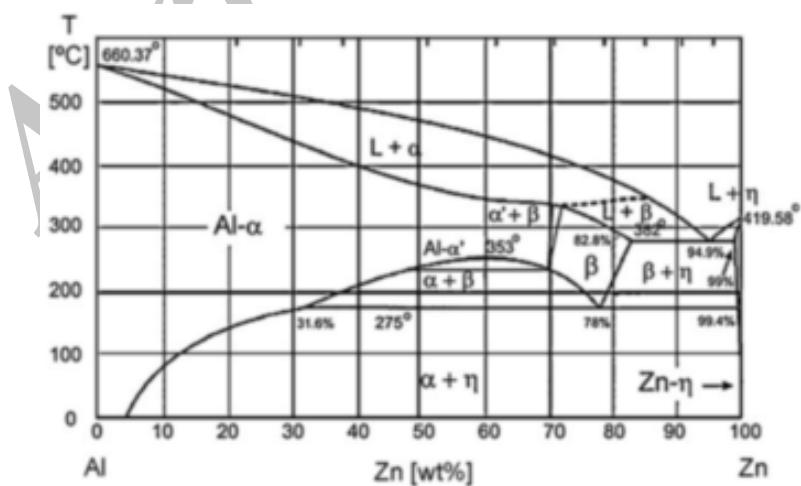
شکل ۶ دیاگرام فازی دوتایی روی-آلومینیم [۱۷]
