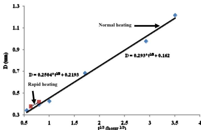
شکل ۷ مقایسه ثابت رشد ذرات در عملیات آنیل القایی و معمولی در 1100^\circ\text{C} درجه سانتیگراد
