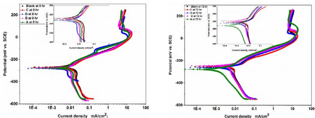
شکل ۵ مقایسه منحنی های پلاریزاسیون پتانسیو دینامیک انواع نمونه ها در محلول 3.5% NaCl در ۰ و ۷۲ ساعت: (الف) ۰ ساعت و (ب) ۷۲ ساعت
