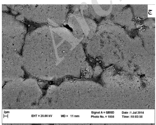
شکل ۲ تصاویر میکروسکوپ الکترونی روبشی کامپوزیت‌های الف - 1.5% Gr - ب - 3% Gr - ج - 4.5% Gr - تولید شده به روش همگن شده در مایع و سپس تفجوشی پلاسمای جرقه‌ای شده
