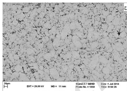
شکل ۱ تصویر میکروسکوپ الکترونی روبشی کامپوزیت های (الف) Al - 1.5 % Gr (ب) Al - 3 % Gr (ج) Al - 4.5 % Gr تولید شده به روش همگن سازی در مایع و سپس پرس سرد-تف جوشی شده
