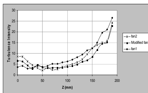
شکل ۱۱ تغییرات شدت اغتشاش برای هر سه فن در محور افقی مرکزی رادیاتور بر حسب فاصله‌ی افقی از مرکز
