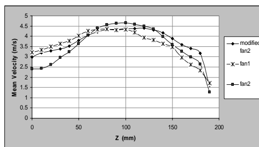
شکل ۱۰ تغییرات سرعت متوسط برای هر سه فن در محور افقی مرکزی رادیاتور بر حسب فاصله‌ی افقی از مرکز
