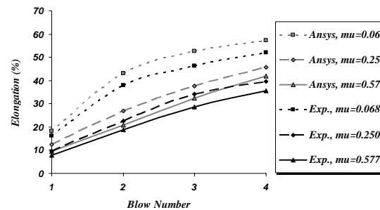
ب) درصد افزایش طول بیلت پس از هر ضربه
