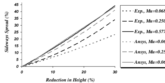
ج) درصد افزایش عرض بیلت در ضربه‌ی اول بر حسب درصد کاهش ارتفاع
