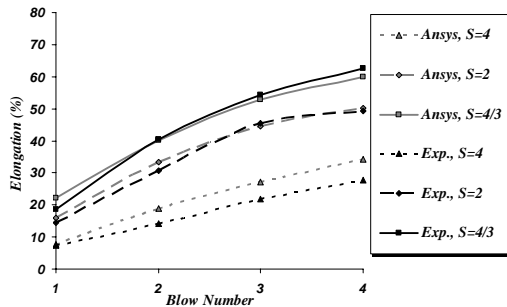
ب) درصد افزایش طول بیلت پس از هر ضربه
