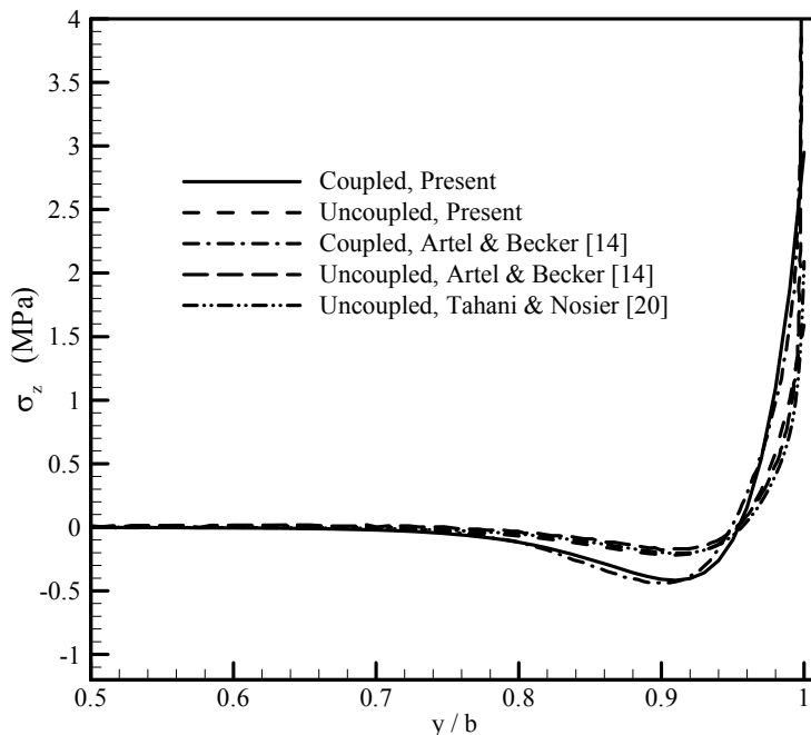
شکل ۲ تنش عمودی بین لایه‌های \sigma_z در چند لایه [0^\circ/90^\circ]_s تحت کرنش یکنواخت محوری در موقعیت z = h/2
