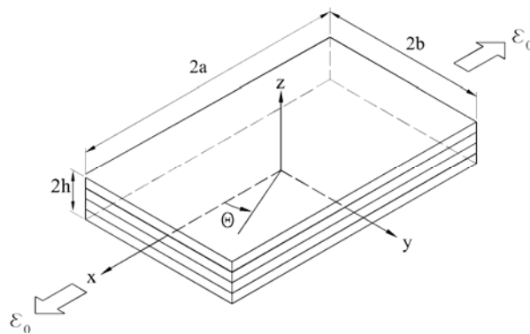
شکل ۱ هندسه و دستگاه مختصات چند لایه‌ی پیزوالکتریک
