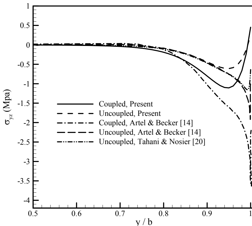
شکل ۴ تنش برشی بین لایه های \sigma_{yz} در چند لایه [0^\circ / 90^\circ]_s تحت کرنش یکنواخت محوری در موقعیت z = h/2
