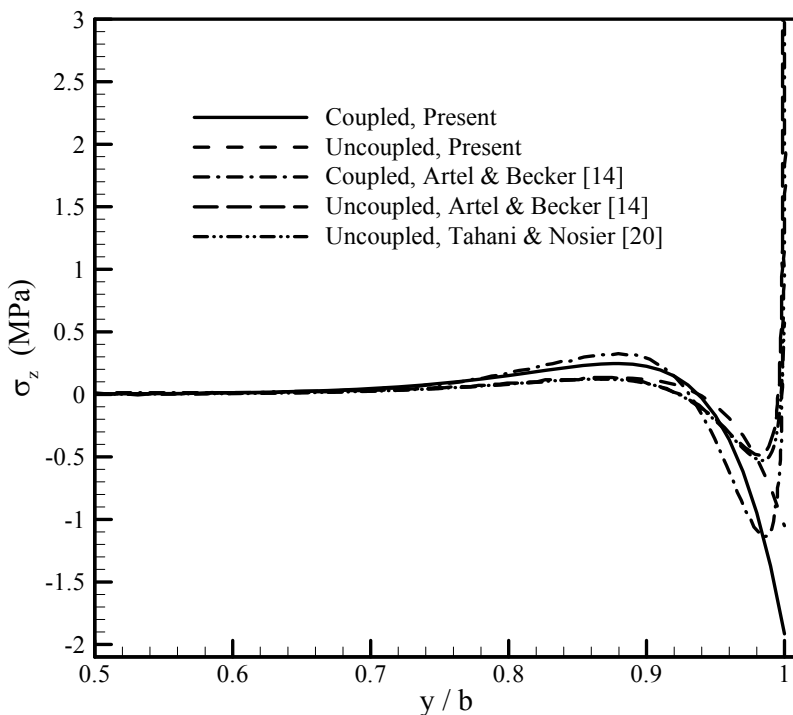
شکل ۳ تنش عمودی بین لایه‌های \sigma_z در چند لایه [90^\circ/0^\circ]_s تحت کرنش یکنواخت محوری در موقعیت z = h/2
