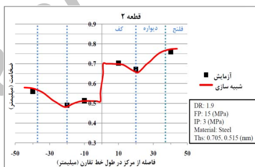
شکل ۲۰ مقایسه‌ی نتیجه‌ی شبیه‌سازی و آزمایش تجربی توزیع ضخامت قطعه‌ی ۲
