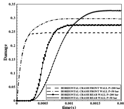
شکل ۱۱ رشد آسیب برای نقطه‌ای در ناحیه‌ی آسیب‌دیده تصادم افقی در سرعت ۱۸۰ km/h و فشارهای متفاوت مخزن
