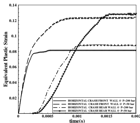
شکل ۱۳ تاریخچه کرنش پلاستیک معادل برای نقطه‌ای در نواحی آسیب‌دیده‌ی تصادم افقی در سرعت ۱۸۰ km/h و فشارهای متفاوت مخزن
