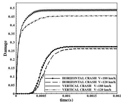
شکل ۲۸ رشد آسیب در نقطه‌ای از ناحیه‌ی آسیب‌دیده‌ی بحرانی برای تصادم در فشارکاری مخزن برای حالت‌های افقی و عمودی
