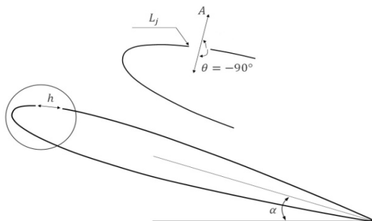
شکل ۱ پارامترهای مکش
