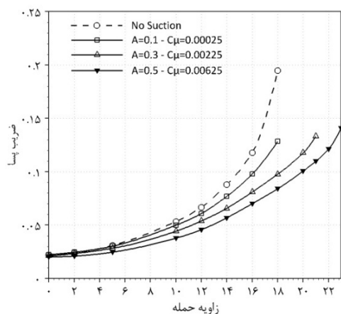
شکل ۹ تأثیر سرعت بی بعد مکش و ضریب مکش بر ضریب پسا در زوایای حمله متفاوت
