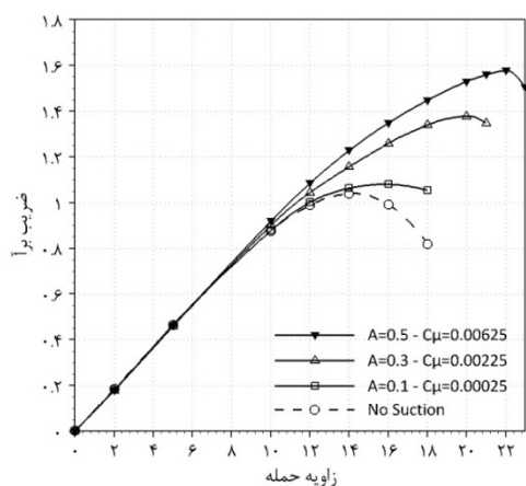
شکل ۸ تأثیر سرعت بی بعد مکش و ضریب مکش بر ضریب برآ در زوایای حمله متفاوت
