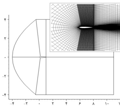
شکل ۲ شبکه‌ی C شکل مش‌بندی شده همراه با بلوک‌بندی
