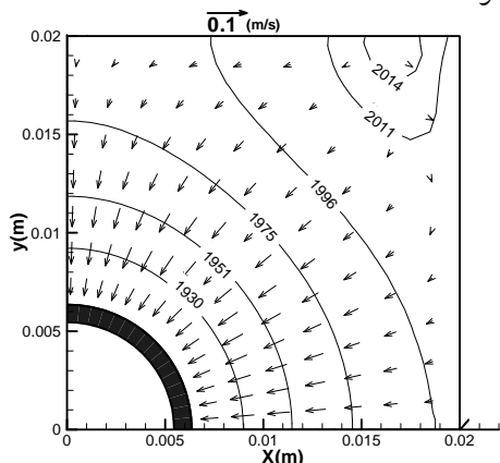
شکل ۷ کانتورهای فشار و بردارهای سرعت در بستر جاذب در صفحه‌ی xy و z=0.05 FS در زمان t=234 sec
