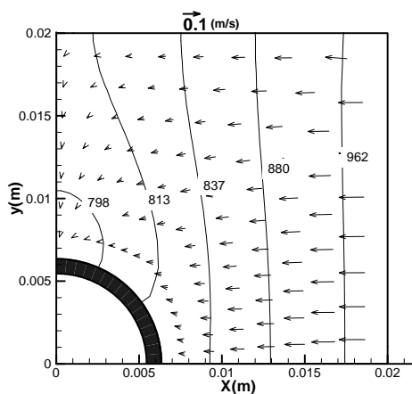
شکل ۸ کانتورهای فشار و بردارهای سرعت در بستر جاذب در صفحه‌ی xy و z=0.05 FS در زمان t=244 sec
