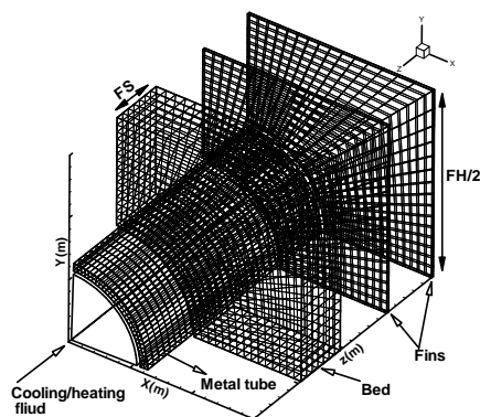
شکل ۳ شبکه‌بندی ۴ حوزه‌ی حل برای مدل‌سازی
