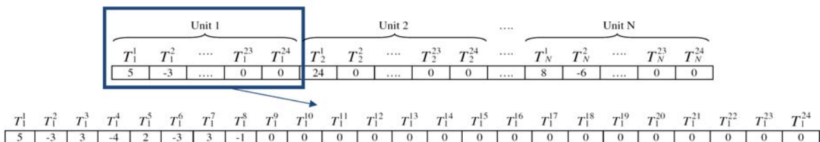
شکل (۲): یک نمونه جواب از جمعیت اولیه شامل وضعیت روشن / خاموش N واحد نیروگاهی طی یک دوره زمانی
