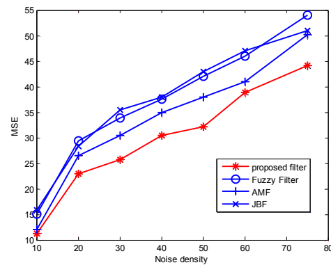
شکل (۶): نمودار میانگین مربع خطای تصویر آنژیوگرافی
