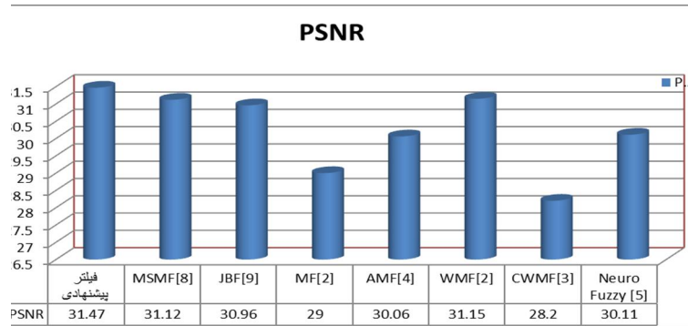
شکل (۵): معیار نسبت نویز به سیگنال فیلترهای حذف نویز
