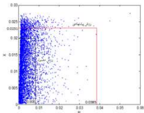
شکل (۱۲): امیدانس دیده‌شده با رله R_1 به ازای خط داخل خط L_1 به همراه تنظیمات روش سنتی و روش پیشنهادی
