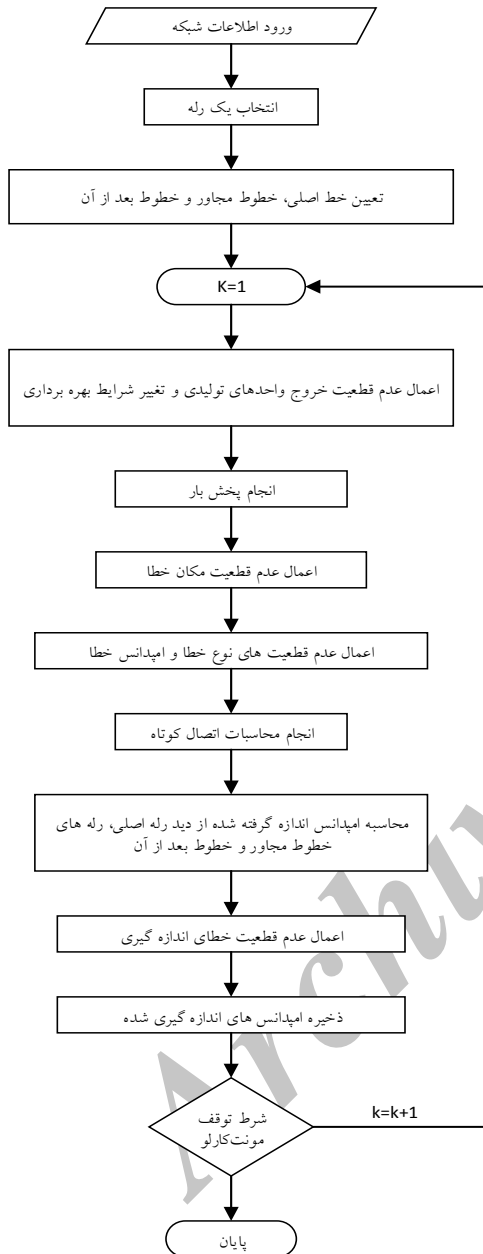
شکل (۲): الگوریتم محاسبه امیدانس‌های اندازه‌گیری شده با رله
