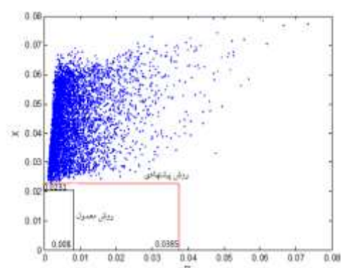
شکل (۱۳): امیدانس دیده‌شده با رله R_1 به ازای خط خارج خط L_1 به همراه تنظیمات روش سنتی و روش پیشنهادی
