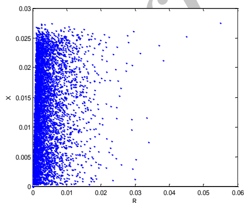
شکل (۵): امیدانس دیده شده با R_1 به ازای خط در خط L_1 با در نظر گرفتن عدم قطعیت‌ها
