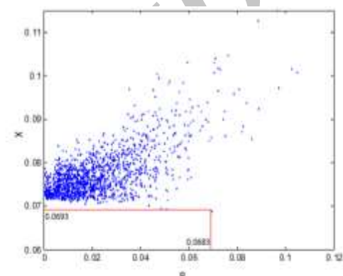
شکل (۱۱): امیدانس دیده‌شده با رله R_1 به ازای خط در خطوط L_{31} و L_{32} و خارج از ناحیه دوم رله R_2 به همراه تنظیم بهینه ناحیه سوم رله R_1
