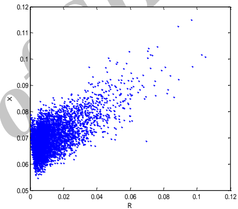
شکل (۷): امیدانس دیده‌شده با R_1 به ازای خط در خطوط L_{31} و L_{32} با در نظر گرفتن عدم قطعیت‌ها
