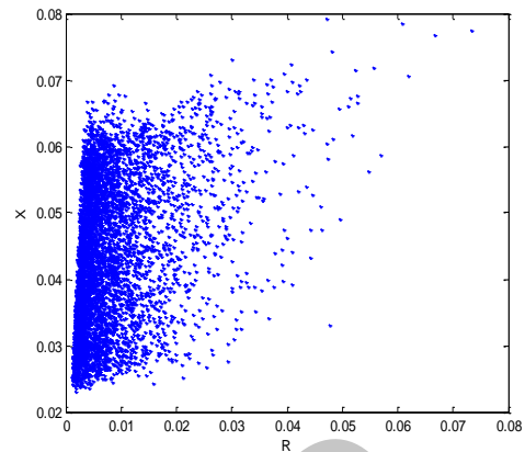
شکل (۶): امیدانس دیده‌شده با R_1 به ازای خط در خط L_2 در نظر گرفتن عدم قطعیت‌ها
