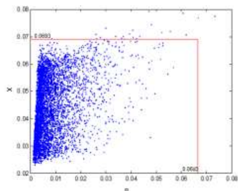
شکل (۱۰): امیدانس دیده‌شده با رله R_1 به ازای خط در خط L_2 به همراه تنظیم بهینه ناحیه سوم رله R_1
