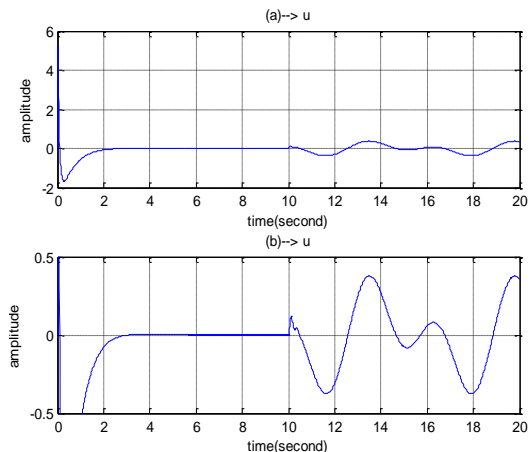
شکل (۶): سیگنال کنترل ورودی موتور
