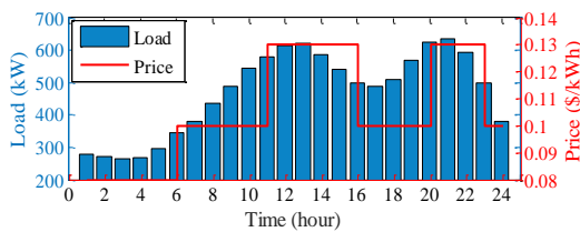
شکل (۴): مقدار پیش‌بینی‌شده بار و قیمت انرژی با تعرفه زمان استفاده (TOU) در افق برنامه‌ریزی [۱].
