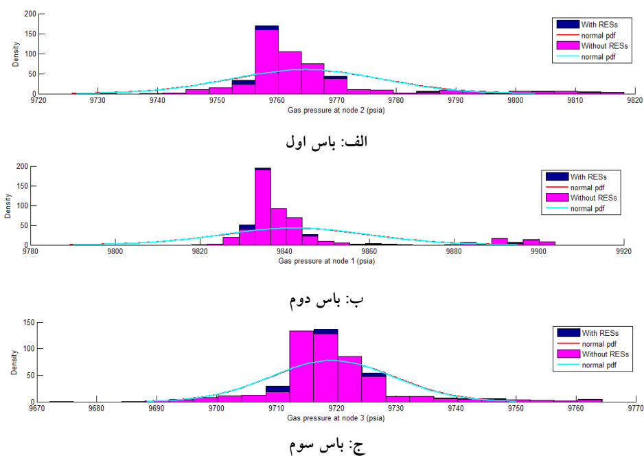
شکل (۸): تابع توزیع فراوانی فشار گاز در باس‌های گازی با و بدون منابع تجدیدپذیر
