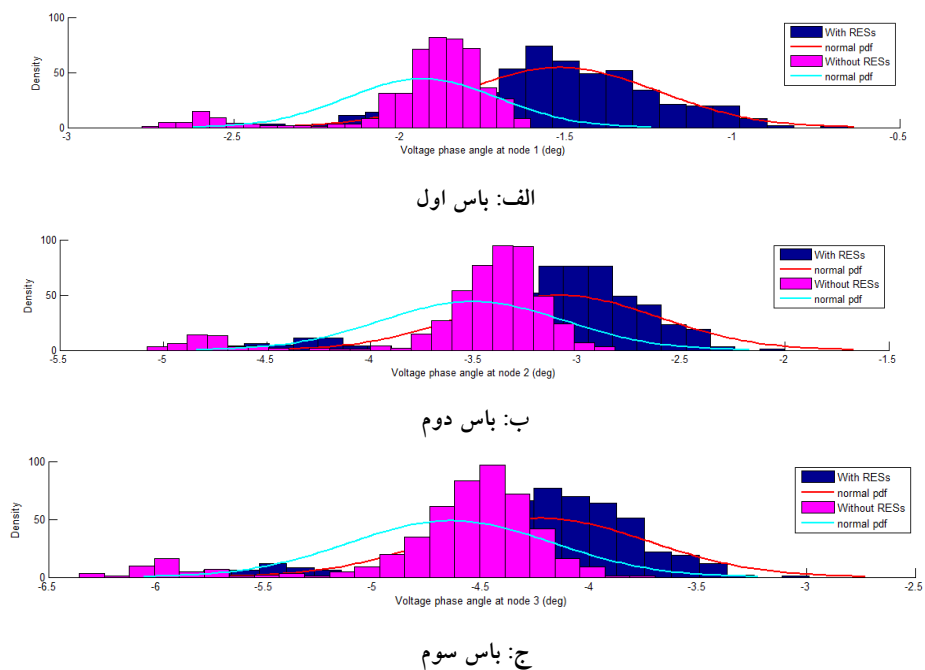
شکل (۷): تابع توزیع فراوانی زاویه فاز در باس‌های الکتریکی با و بدون منابع تجدیدپذیر
