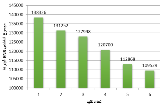
شکل (۹): مجموع شاخص ENS فیدرها برحسب تعداد کلیدها با در نظر گرفتن اهمیت یکسان برای فیدرها و باوجود تولید پراکنده در فیدر متصل به بار AL 23
