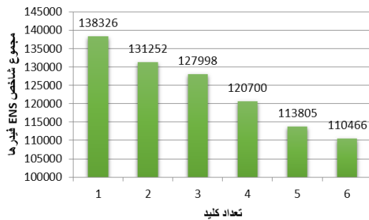
شکل (۷): مجموع شاخص ENS فیدرها برحسب تعداد کلیدها با در نظر گرفتن اهمیت یکسان برای فیدرها و بدون تولید پراکنده
