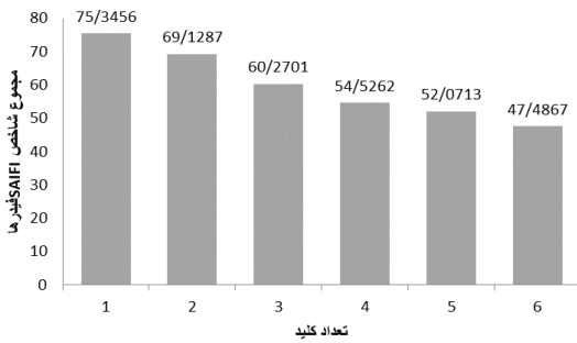
شکل (۶): مجموع شاخص SAIFI فیدرها برحسب تعداد کلیدها با در نظر گرفتن اهمیت یکسان برای فیدرها و بدون تولید پراکنده
