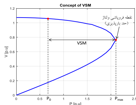
شکل (۷): مفهوم حد پایداری و لتناژ
