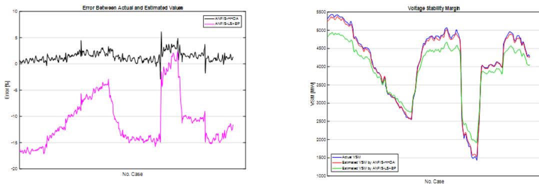
شکل (۱۲): خطای نرمالیزه شده تخمین VSM به کمک ANFIS-LS+BP و ANFIS-HHOA
