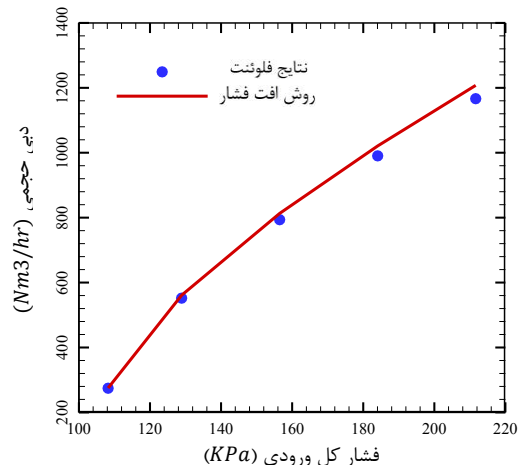
شکل ۱۰- مقادیر دبی حجمی شاخه‌های شماره ۱ و ۲ شبکه مربوطه
