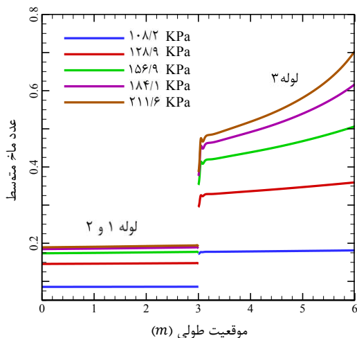
شکل ۸- تغییرات عدد ماخ متوسط در راستای طول انشعاب‌ها به ازای فشارهای مختلف ورودی
