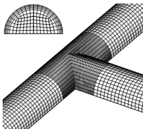
شکل ۲- نمایی از شبکه با سازمان اتصال مورد نظر و نمای برش خورده از سطح مقطع آن
