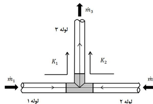
شکل ۱- اتصال T- شکل مورد نظر
